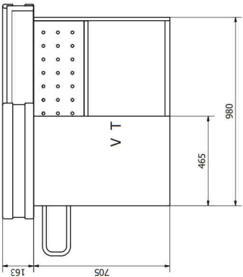
SIDE ELE A ION ( 1 : 10 )
