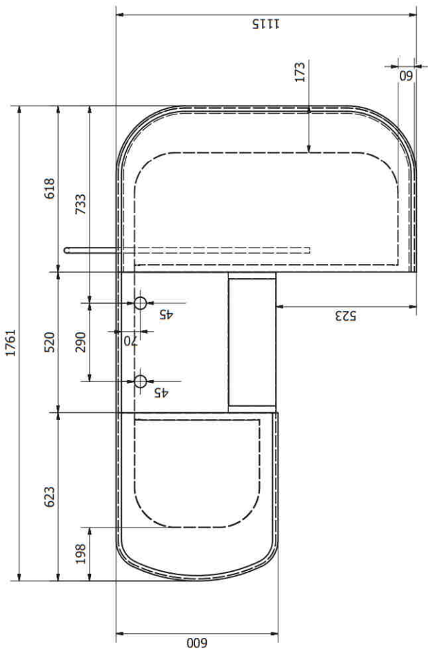
TOP ELEVATION ( 1 : 10 )
