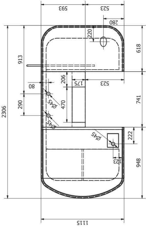
TOP ELEVATION ( 1 : 15 )
